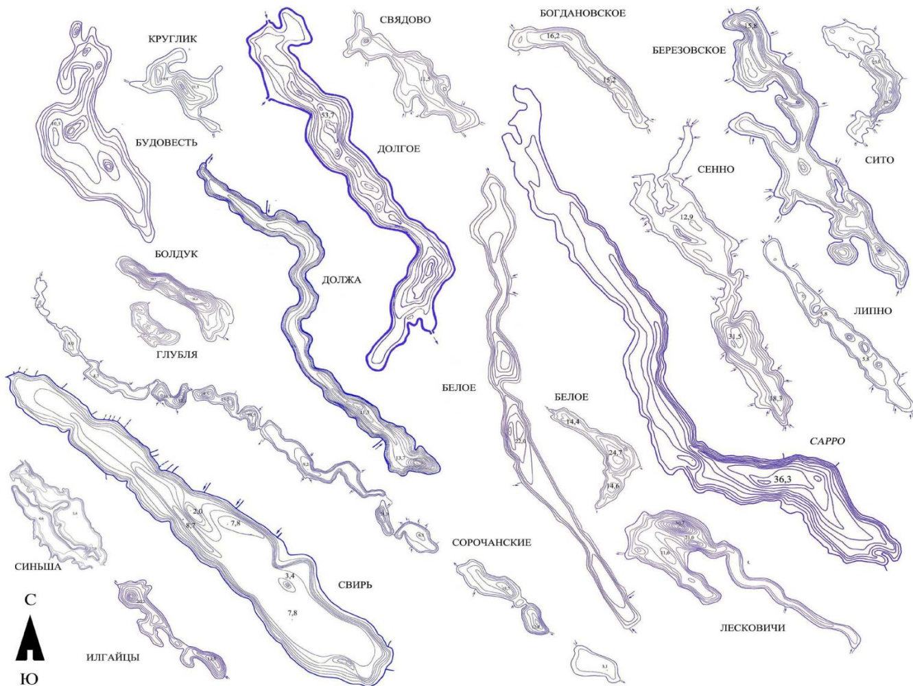
Схема ориентации ложбинных озер Белорусского Поозерья (по Новику А.А.).
