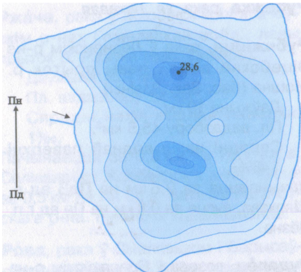
Батимметрическая схема озера эвразийного типа (оз.Рудаково)
